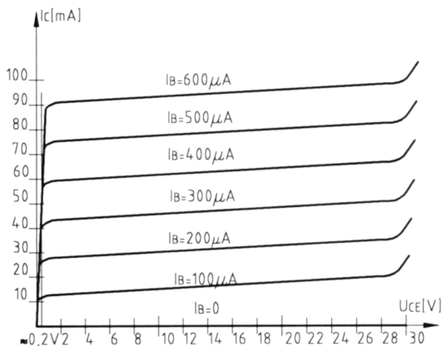
32. ábra Szilícium npn tranzisztor U_{CE} - I_C karakterisztikája
