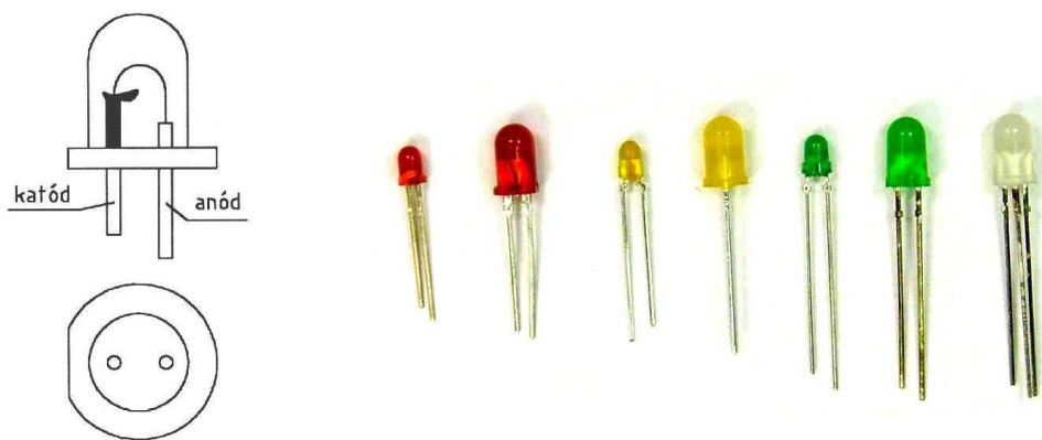
27. ábra LED és bekötése
