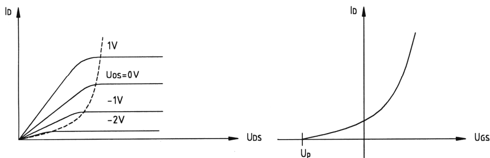
43. ábra Kiürítéses MOS FET karakterisztikái
