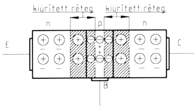
28. ábra n-p-n tranzisztor feszültségmentes állapotban
