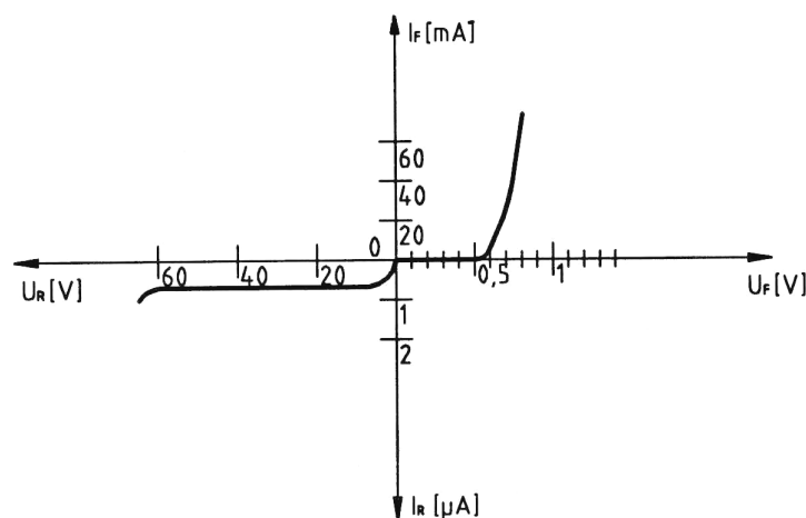
16. ábra Si dióda karakterisztikája
