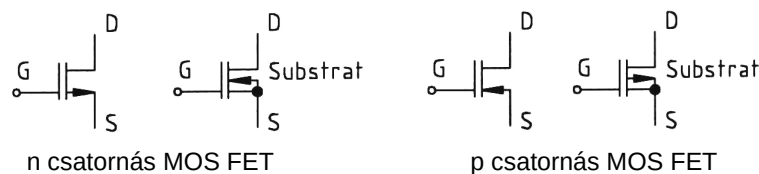
46. ábra MOS-FET áramköri rajzjelei
