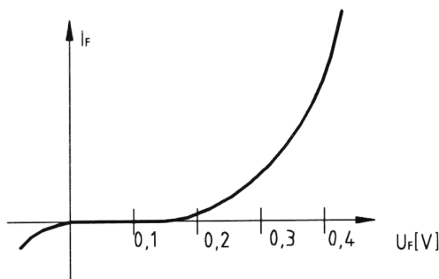
24. ábra Schottky-dióda karakterisztikája
