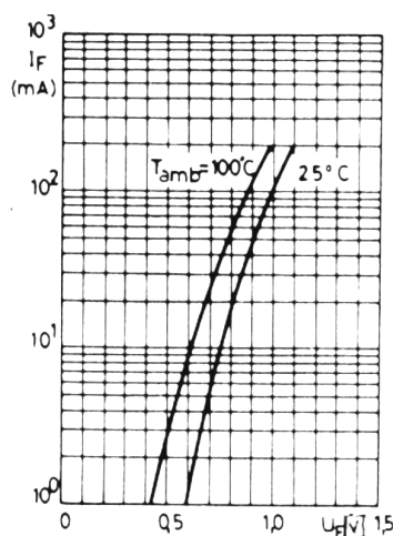
17. ábra Az 1N4151 dióda nyitóáramának hőfokfüggése
