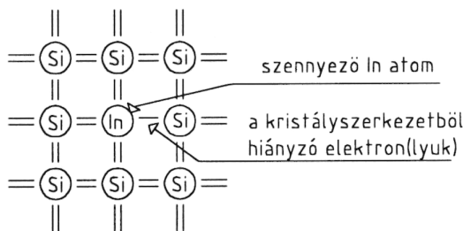
6. ábra „p” típusú Si előállítás In akceptorszennyezéssel
