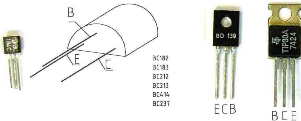
34. ábra Tranzisztorok kivezetéseinek bekötése
