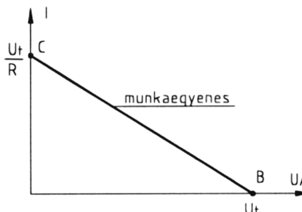
b) Munkaegyenes
