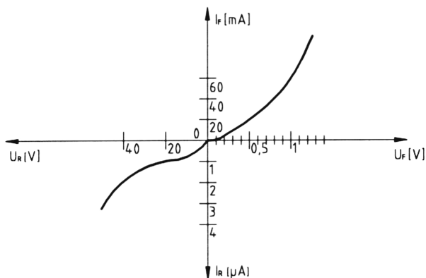
14. ábra Ge dióda karakterisztikája
