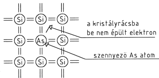
5. ábra „n” típusú Si előállítás As donorszennyezéssel
