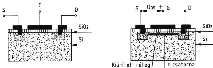
44. ábra n csatornás növekményes MOS FET kialakítása
