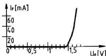
25. ábra Vörös (GaAsP) LED nyitókarakterisztikája, és a LED áramköri rajzjele
