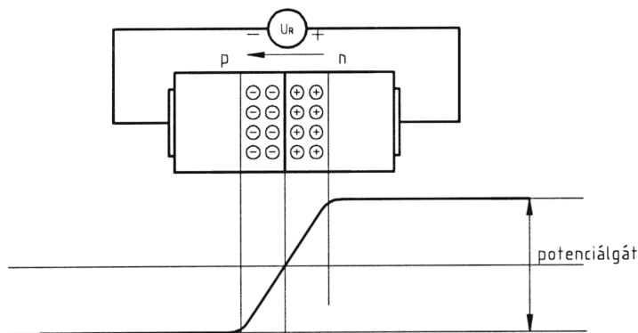
9. ábra Záró irányban előfeszített dióda
