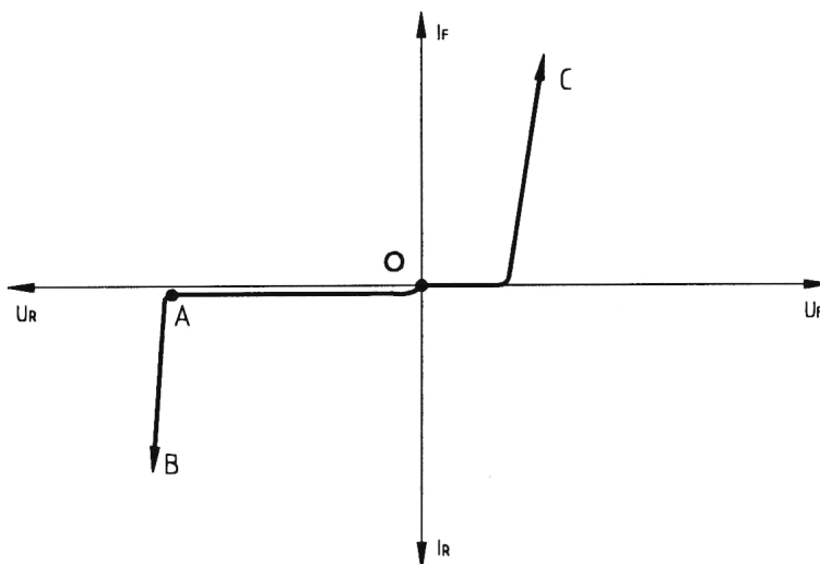
10. ábra A dióda karakterisztikája
