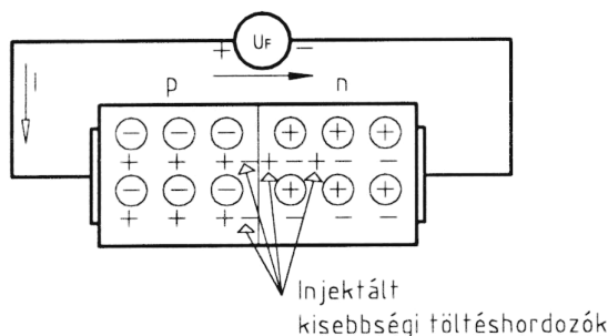
11. ábra Nyitóirányban előfeszített dióda
