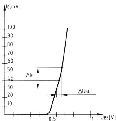
31. ábra Szilícium npn tranzisztor U_{BE} - I_E karakterisztikája
