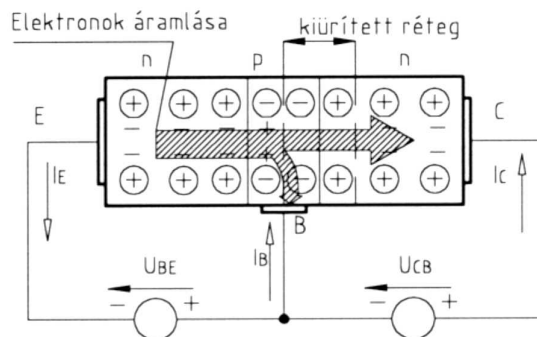
29. ábra n-p-n tranzisztor előfeszített állapotban
