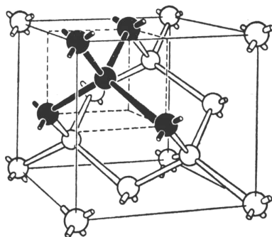
a) Szilíciumkristály
