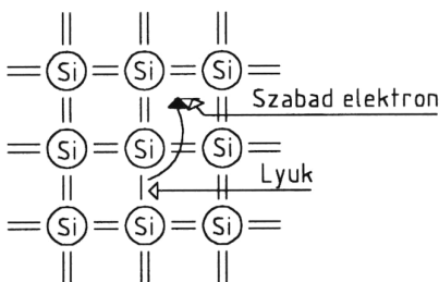
2. ábra Szabad elektron - lyuk páros keletkezése
