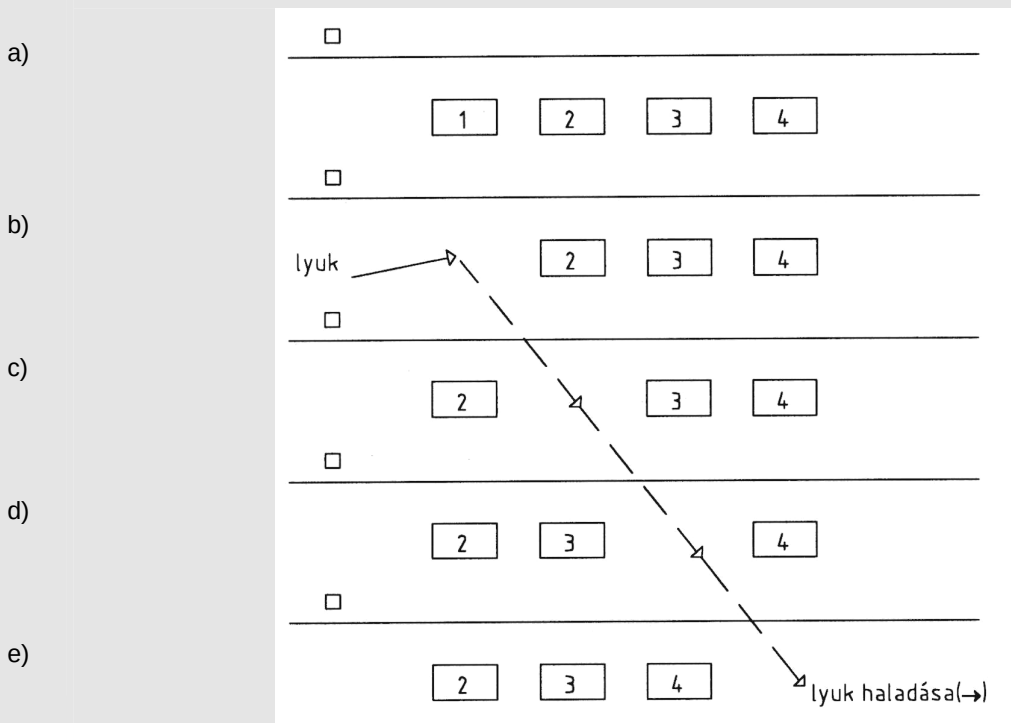
4. ábra „Lyukvezetés” taxikkal szemlélítve
