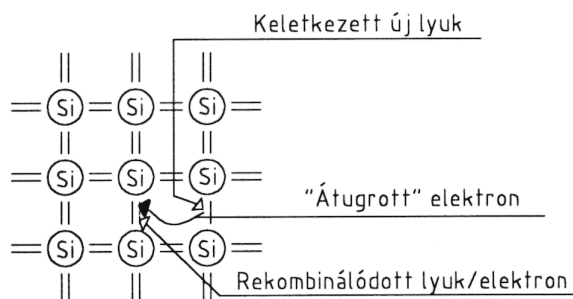
3. ábra Lyukvezetés
