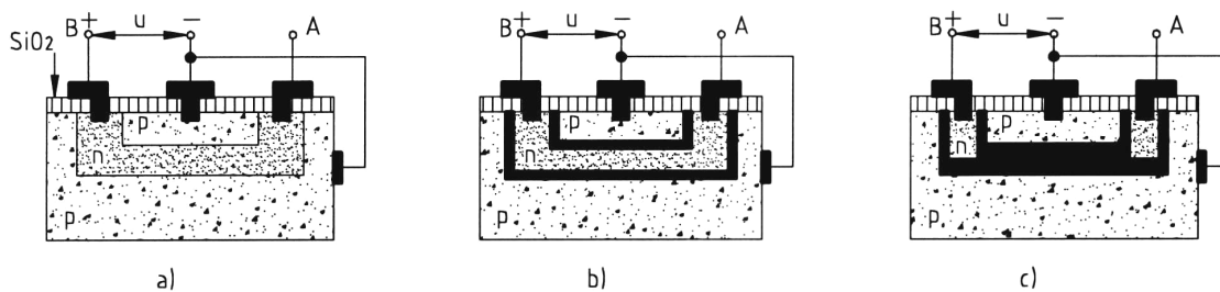
38. ábra Feszültséggel vezérelhető ellenállás
