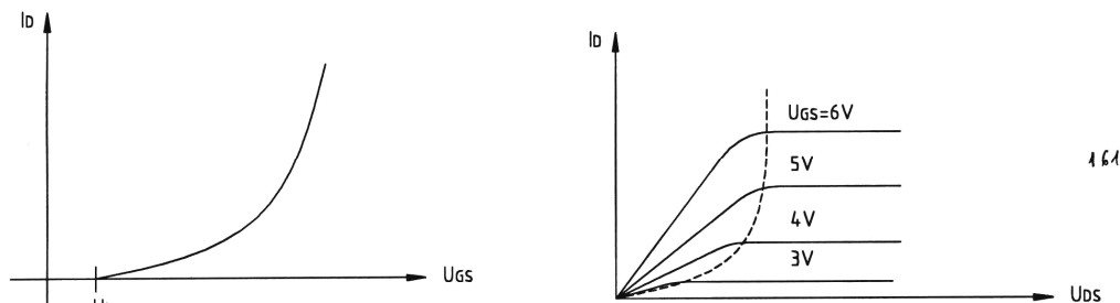
45. ábra Növekményes MOS FET karakterisztikái
