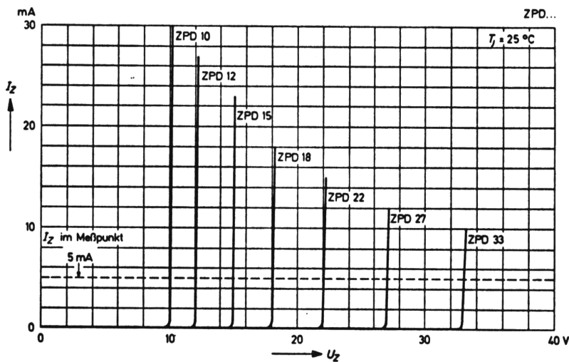
19. ábra ZPD sorozat karakterisztikái
