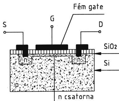
42. ábra Kiürítéses üzemmódú MOS FET
