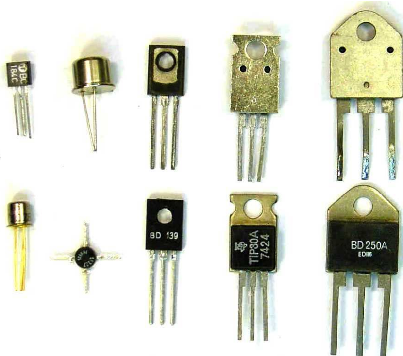
33. ábra Kis és közepes teljesítményű tranzisztorok
