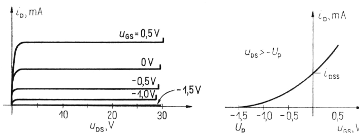
41. ábra n csatornás JFET karakterisztikái
